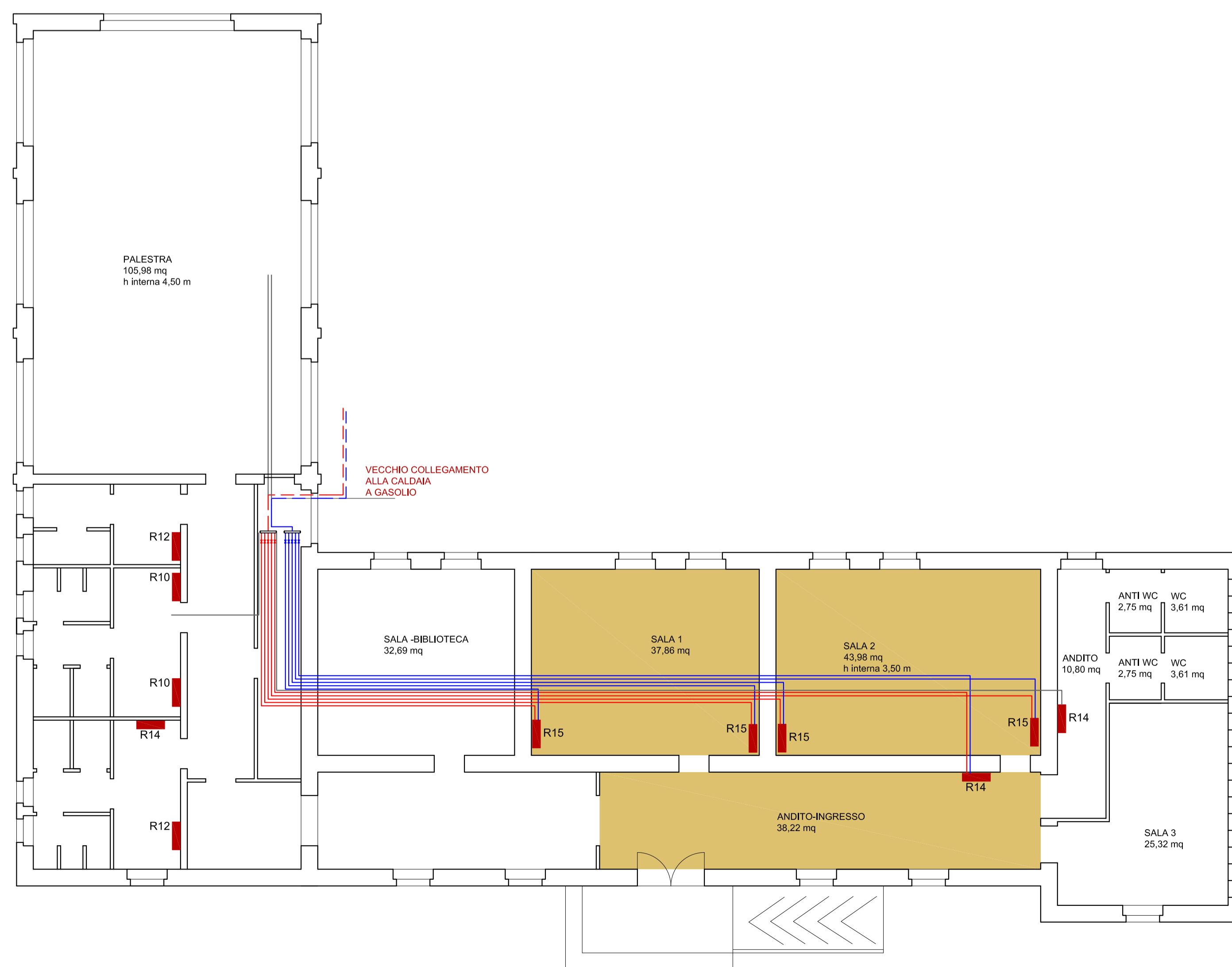
Pianta con individuazione dei radiatori esistenti
